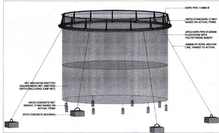
ELEVATION SCALE: NTS
