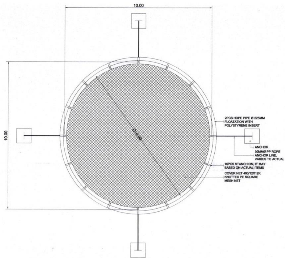
TOP VIEW SCALE: 1: 100 MTS
