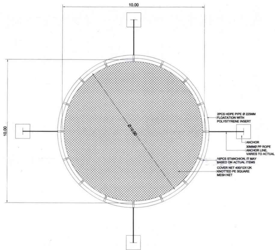
TOP VIEW SCALE: 1: 100 MTS
