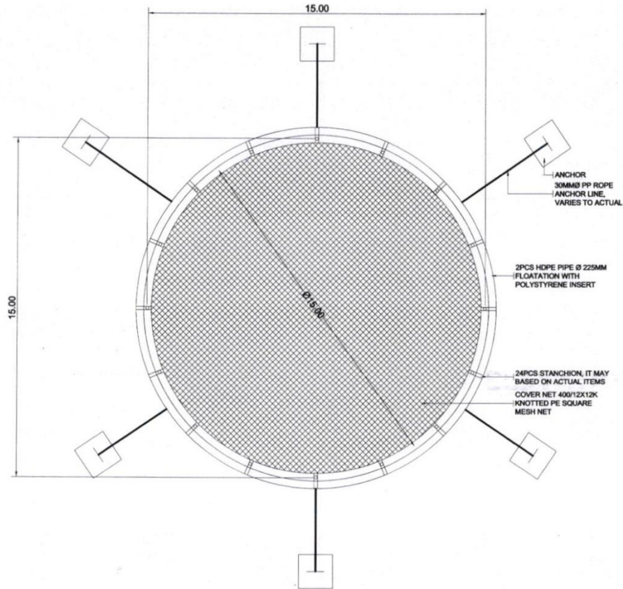
TOP VIEW SCALE: 1: 100 MTS
